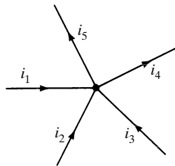
Figure 6-5 Node. i_1 + i_2 + i_3 - i_4 - i_5 = 0 .
